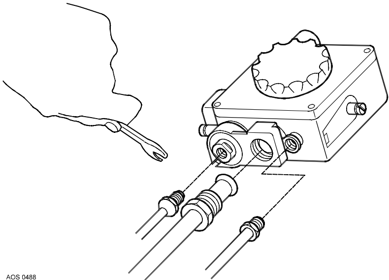
Desenho 11 - Montagem do conjunto de queimador
