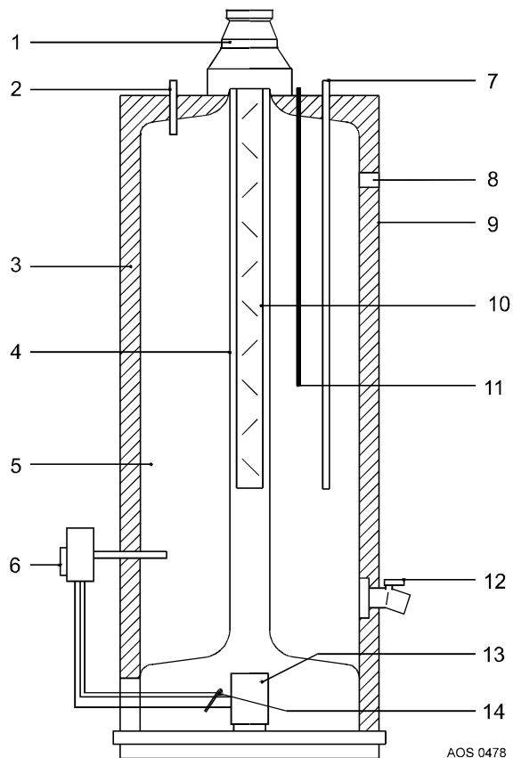
Desenho 1 - corte longitudinal do aparelho
