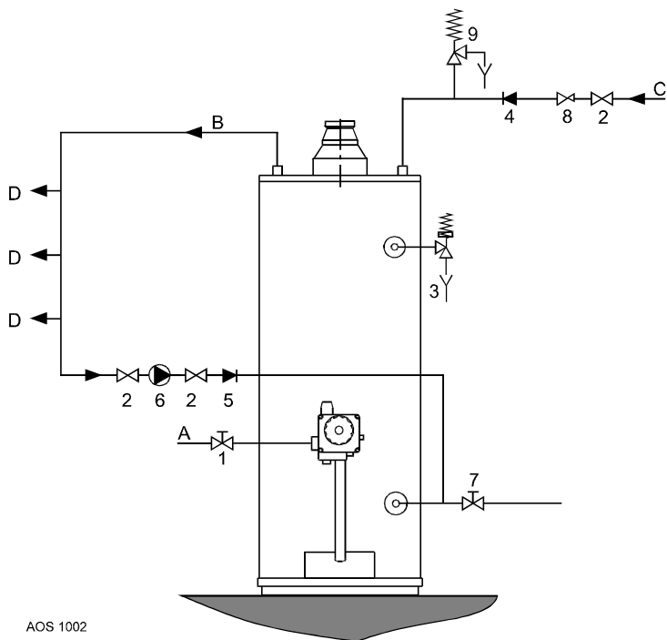
Desenho 4 - Esquema de ligação
