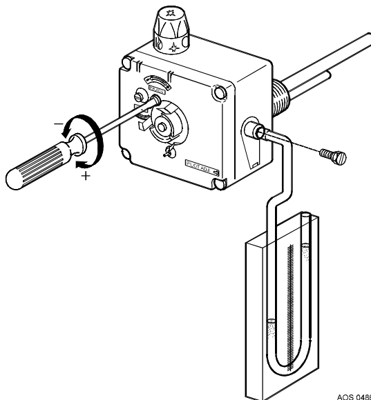
Desenho 9 - Regulagem da capacidade nominal
