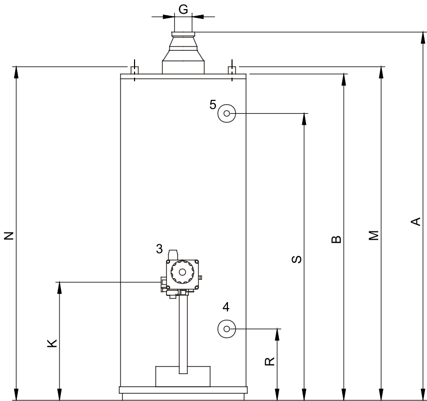
Desenho 3 - Dimensões
