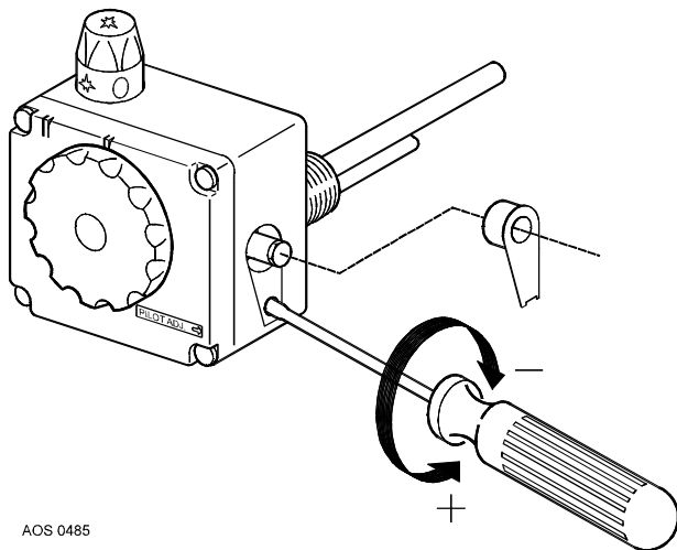
Desenho 8 - Regulagem da chama-piloto
