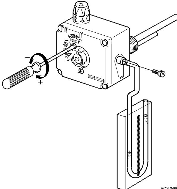
Abbildung 9 - Einstellen der nominalen Belastung
