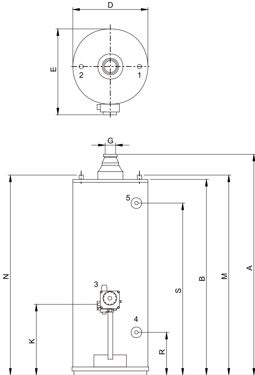
Abbildung 3 - Abmessungen
