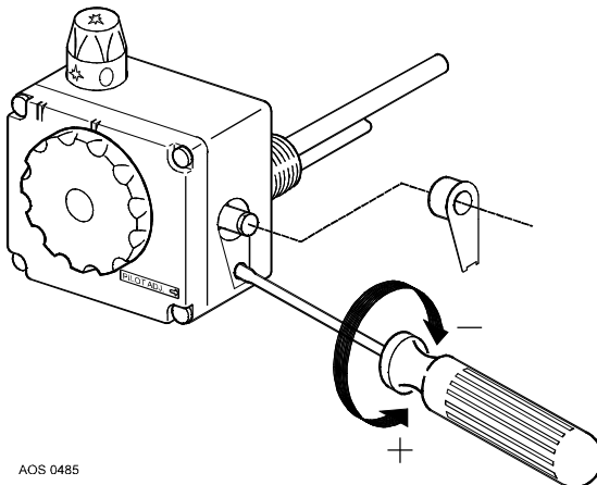
Abbildung 8 - Einstellen der Wachflamme
