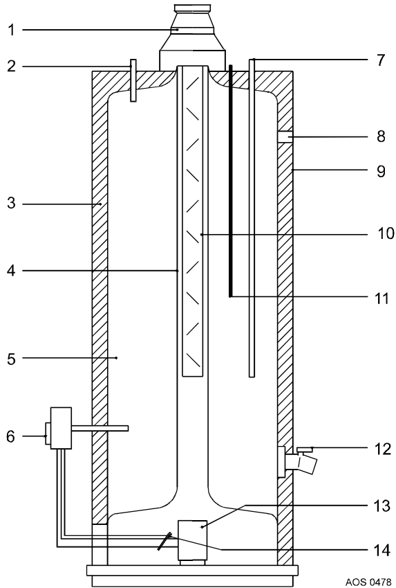
Abbildung 1 - Querschnitt durch das Gerät
