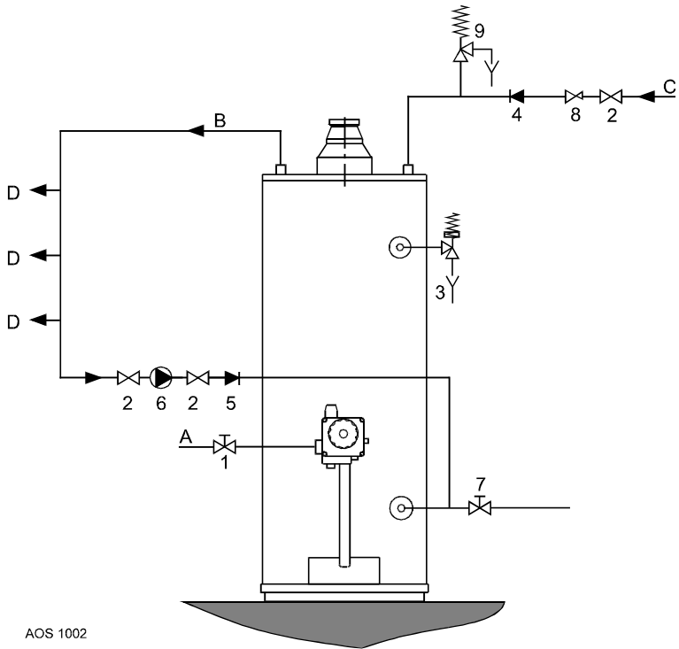
Abbildung 4 - Anschlußplan
